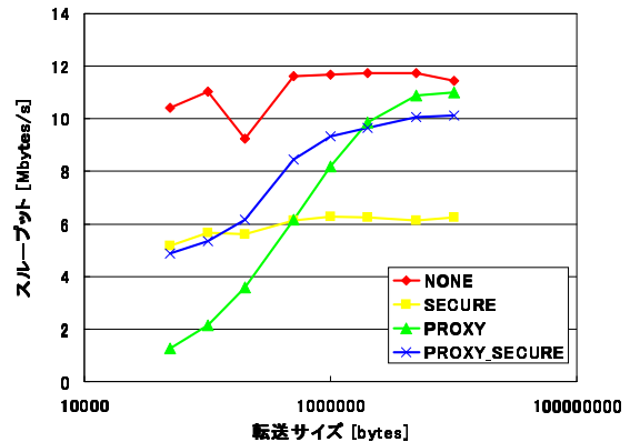
図 9 100base/TX での実験
