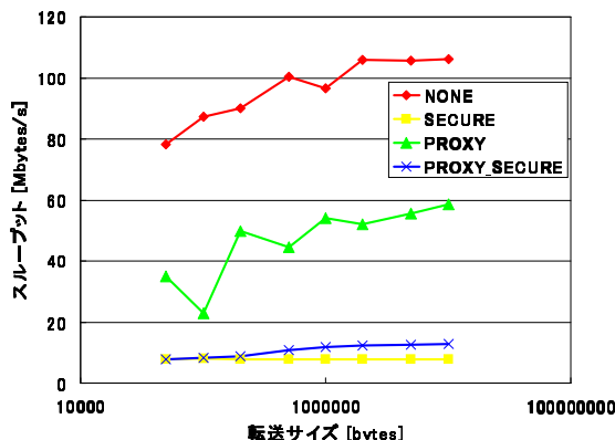
図 10 1000base/T での実験
