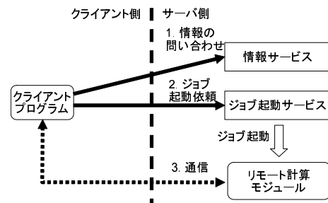
図1 Ninf-G の概要
