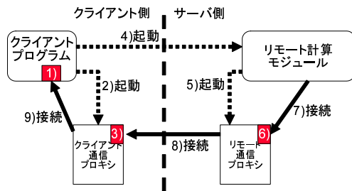
図 5 通信プロキシによる通信路の確立
