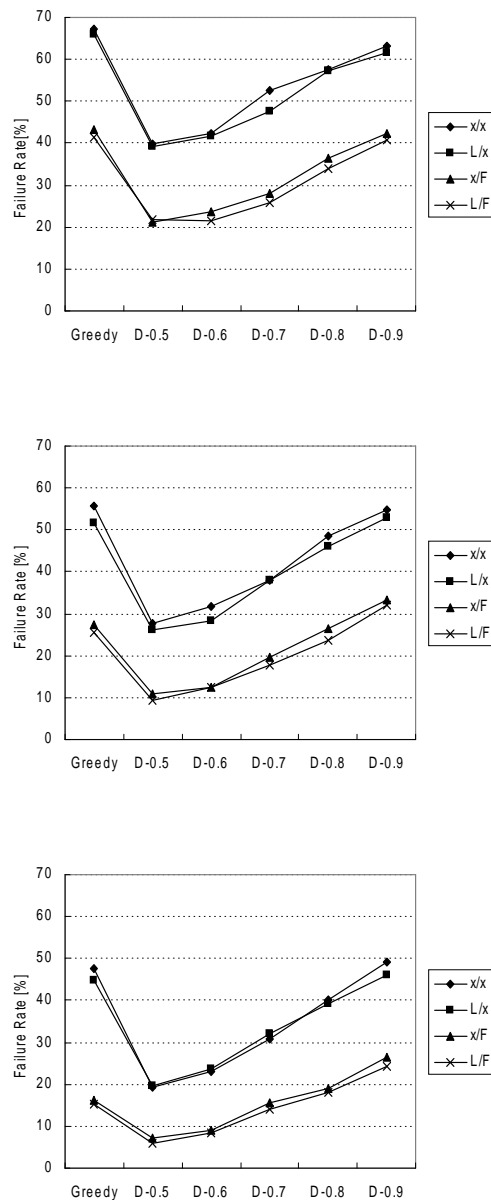
図3 Greedy と Deadline のスケジューリング失敗率の比較 ( N_{max. fallbacks} = 1 , Int=60 (上), 90 (中), 120 (下))。
